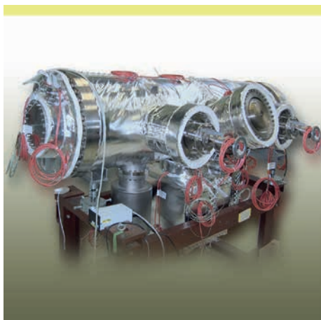
Beheizter Vakuumrezipient
